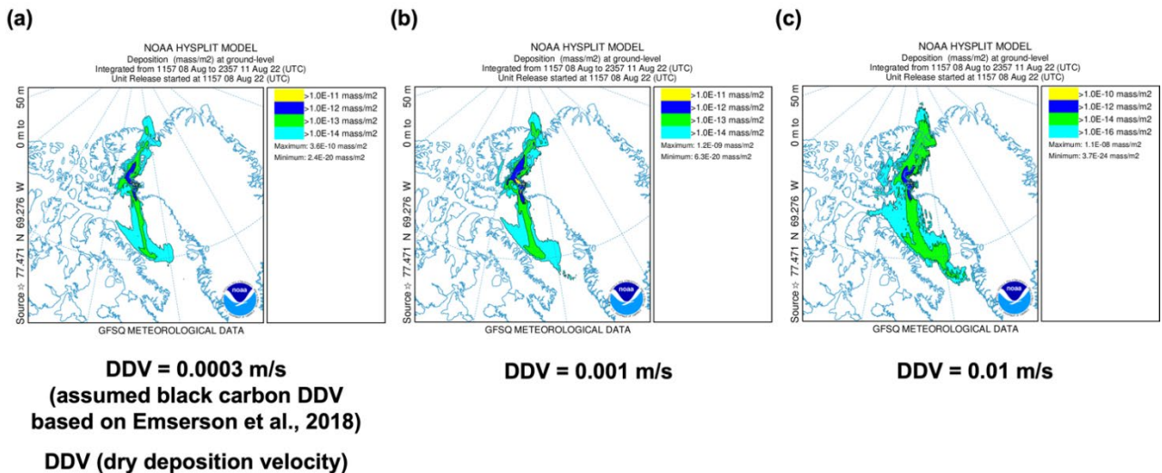
図 3. NOAA HYSPLIT モデルを用いた、三つの異なる乾性沈着速度 (DDV) によるカナックのゴミ置き場の地点からの粒子拡散による相対累積沈着量の計算：(a) DDV = 0.0003 \text{ m s}^{-1} (Emerson et al., 2018) によるブラックカーボンを想定した乾性沈着速度に基づく)；(b) DDV = 0.001 \text{ m s}^{-1} ；(c) DDV = 0.01 \text{ m s}^{-1} 。3.5 日間の前方拡散計算は、2022 年 8 月 8 日 11 時 57 分 (UTC) に開始した (図 2a の現地時間 9 時 57 分に基づく)。
